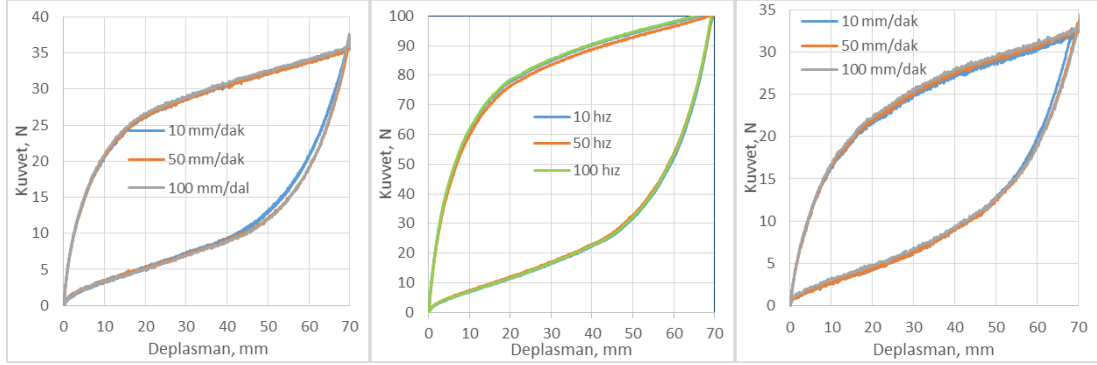
Şekil 4.3. Sırasıyla NÇHTİ, PÇHTİ, GÇHTİ yuvarlanma yük-deplasman cevapları
