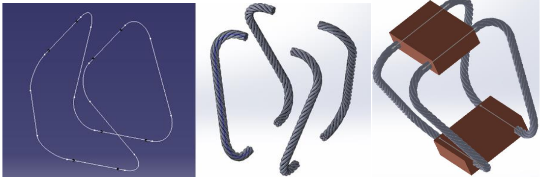
Şekil 2.2. ÇHTİ katı modelinin oluşturulması
