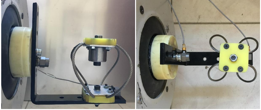
Şekil 3.14. NÇHTİ, PÇHTİ ve GÇHTİ dikey yöndeki titreşim testleri
