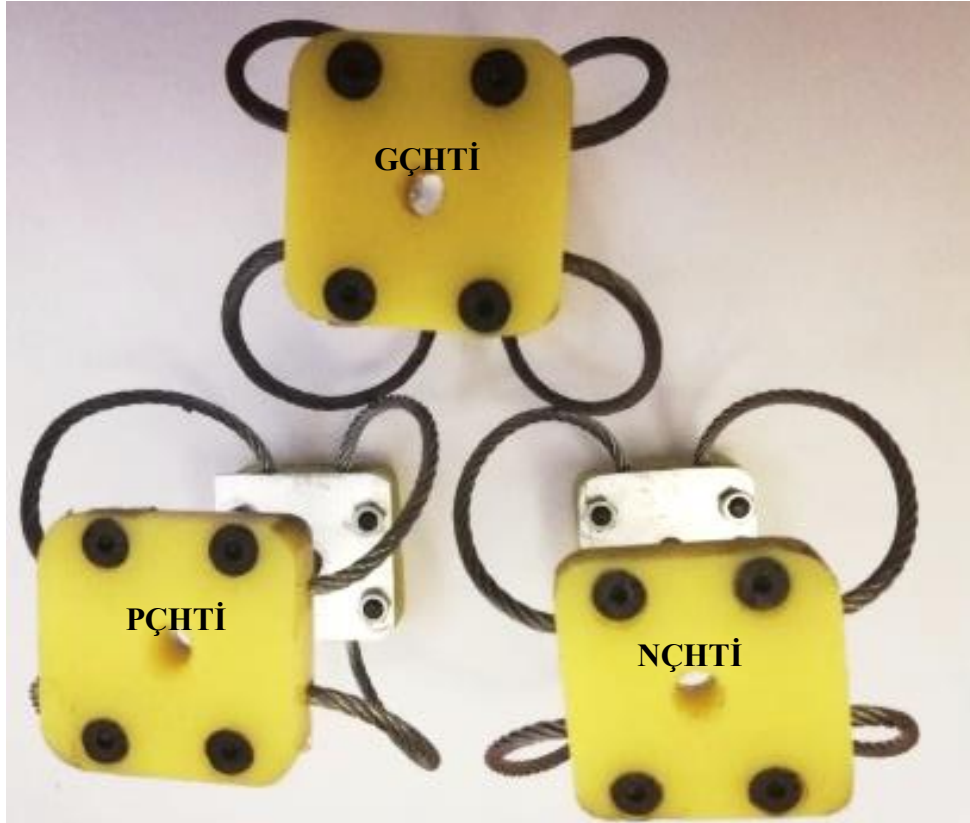
Şekil 2.10. Telleri S şeklinde burarak montajlama
